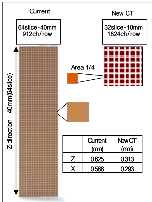
第 3 図 検出器の新旧比較
