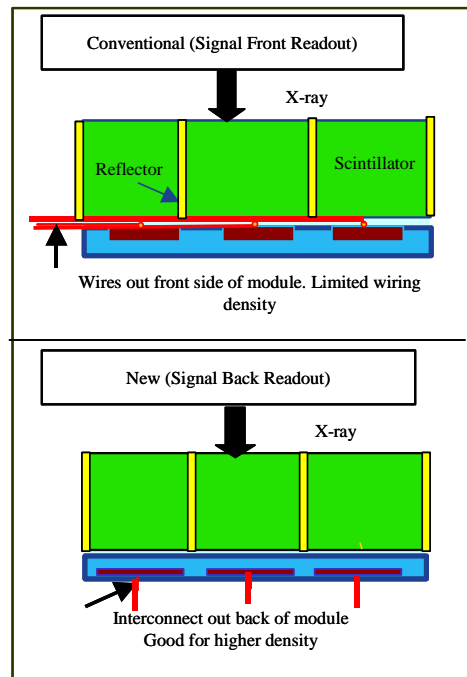
第 4 図 検出器信号取り出し方法の新旧比較
