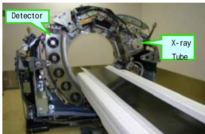
第6図 新CTシステムの外観
