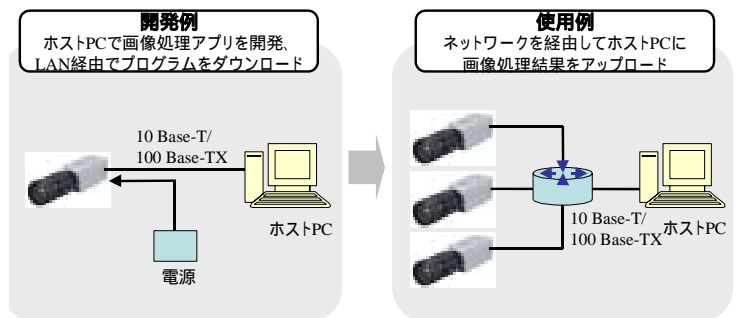
第 4 図 ネットワークシステム
