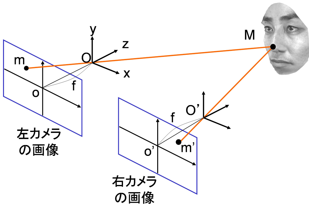
第1図 ステレオビジョンによる3次元計測
