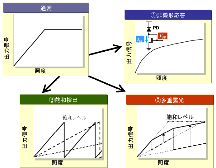
第 3 図 広ダイナミックレンジ手法
