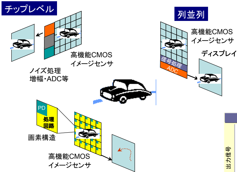
第 1 図 インテリジェントイメージセンサの方式
