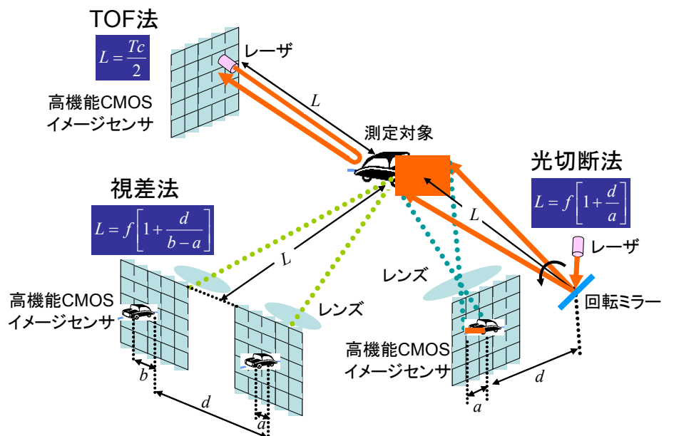
第 5 図 3次元距離計測法
