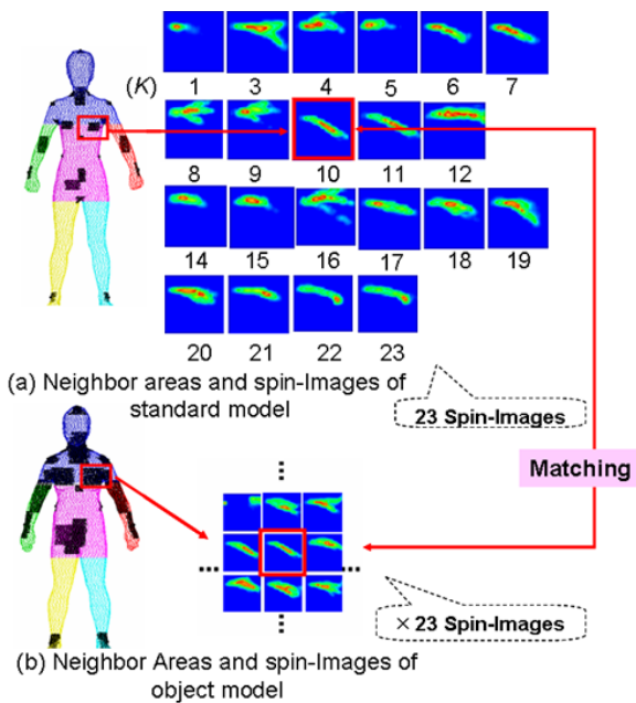
第 4 図 スピンイメージのマッチングの例
