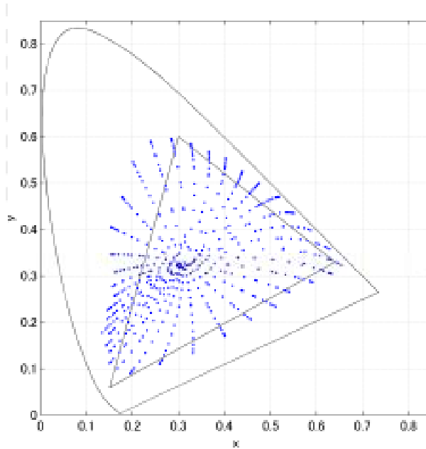
第 1 図 ディスプレイの広色域化
