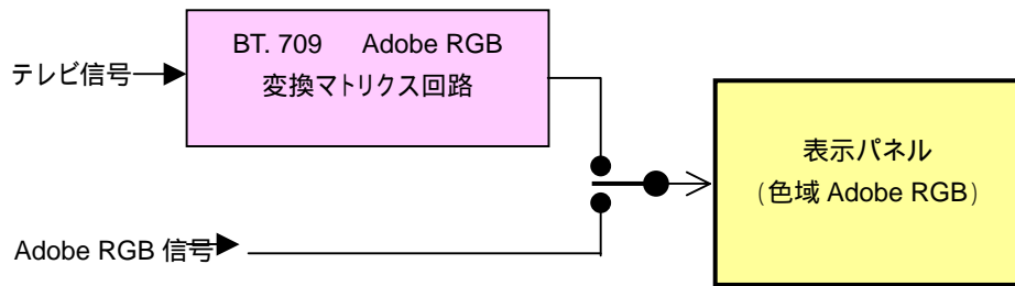
第 2 図 テレビ信号に対応した広色域ディスプレイの例
