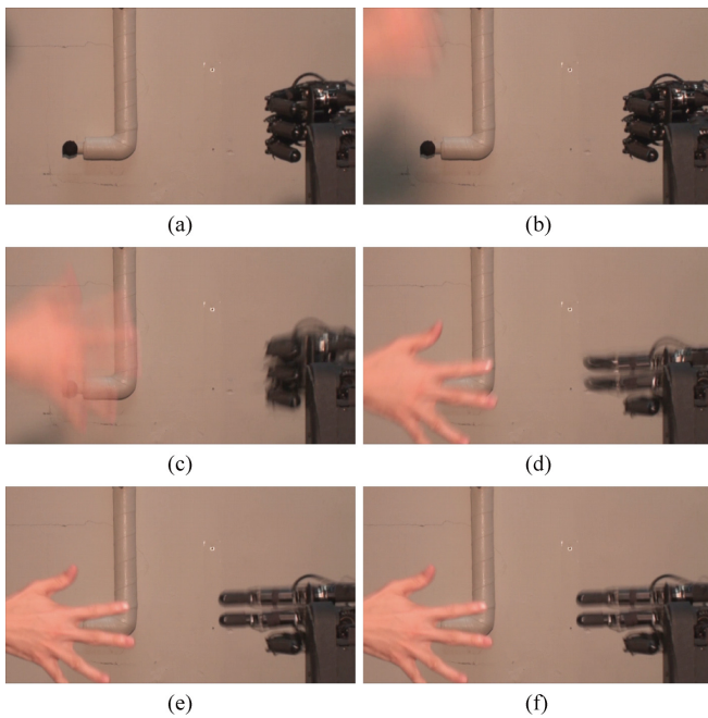
第5図 じゃんけんロボットの実験結果
