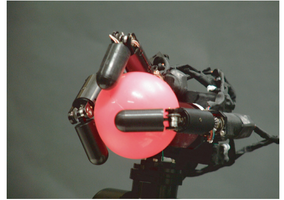
第3図 高速ロボットハンド
