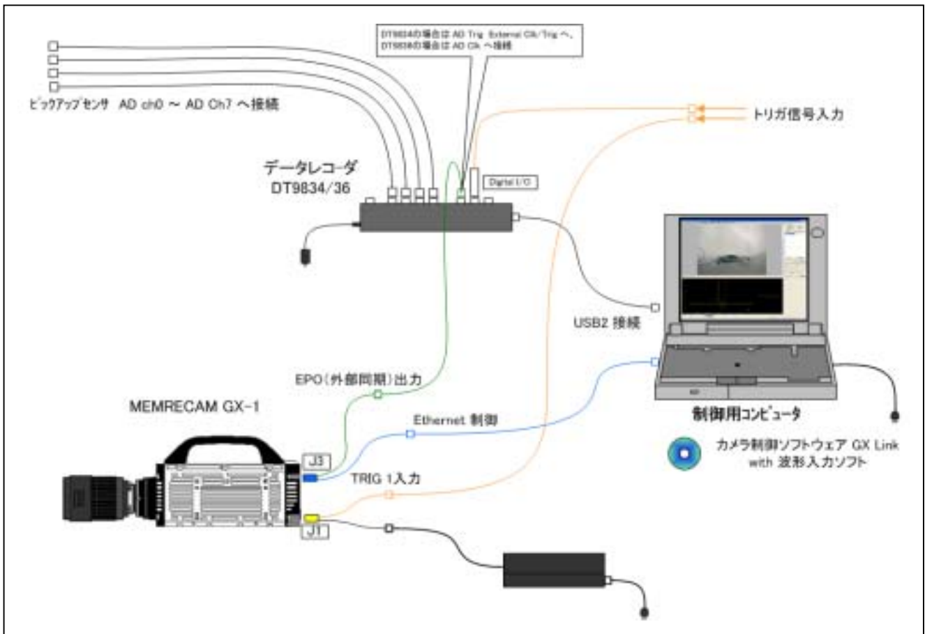
第2図 同期収録システム構築例
