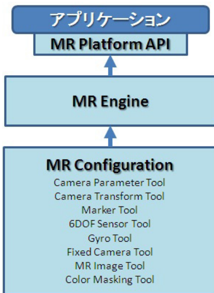
第3図 新たな MR プラットフォームの構成
