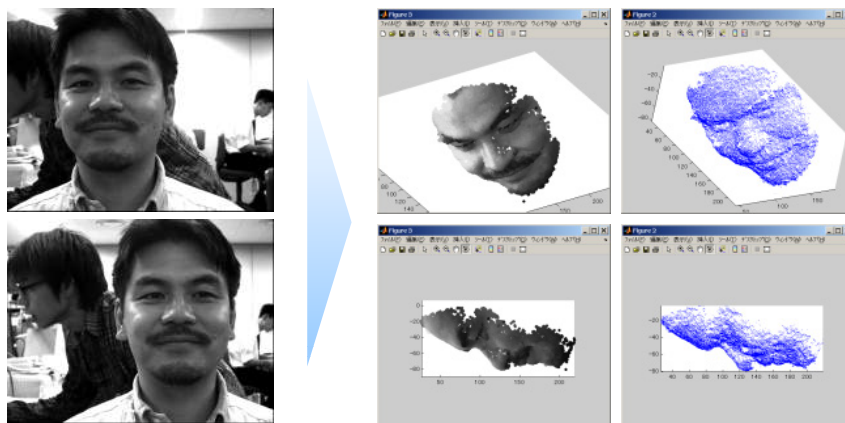
第3図 ステレオ画像と3D顔データ (上段:位置ずれた2枚の画像, 中段:位相限定相関関数, 下段:相関ピークモデルのフィッティングによるサブピクセル移動量推定)
