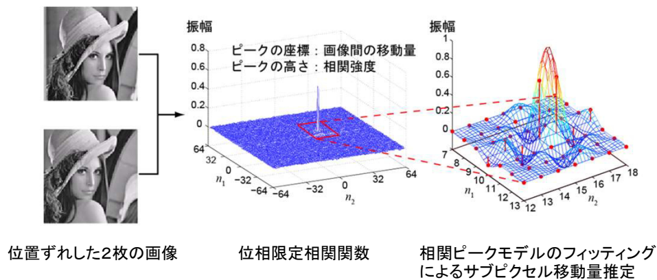
第2図 位相限定相関法
