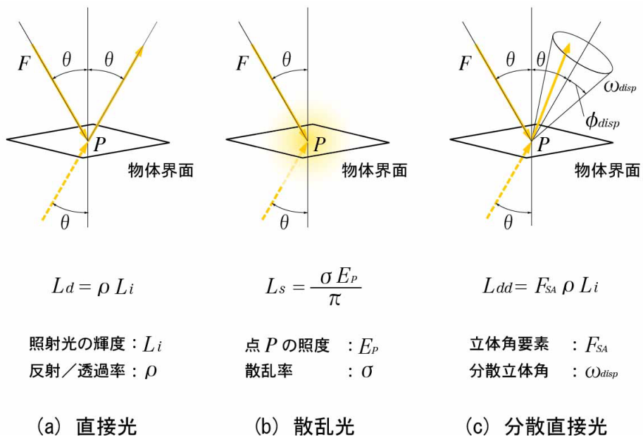
第6図 物体界面における光の伝搬方向の変化と輝度
