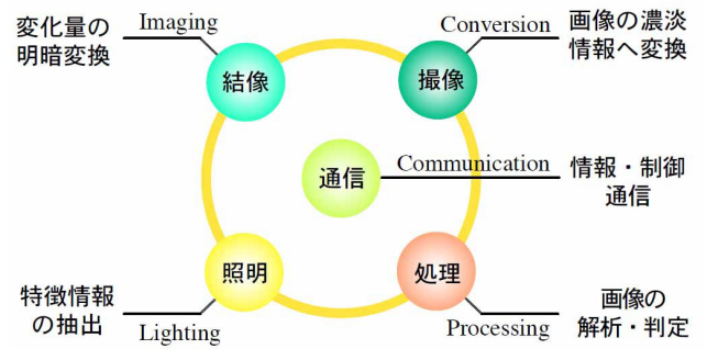
第3図 ビジョンシステムの機能要素
