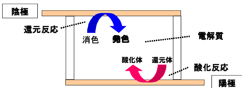
第1図 典型的なECセルの構成と発色機構
