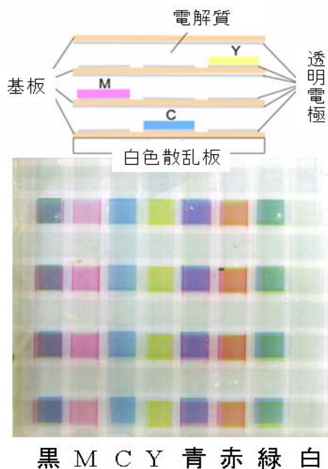
第3図 発色状態にある CMY 三色積層型 EC セル
