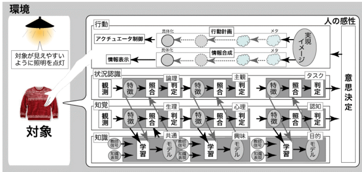
第1図 ロボティクスの枠組みによる感性のモデル表現
