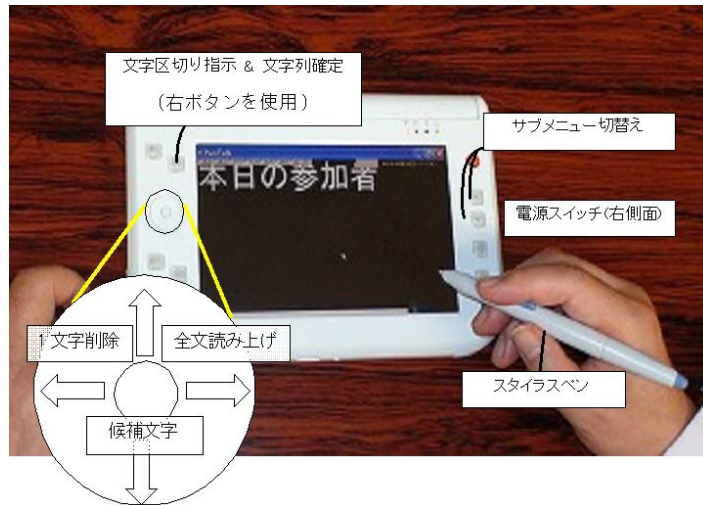
第1図 “Pen-Talker”の概観とコマンドのボタン配置
