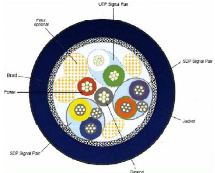
第1図 USBケーブルの芯線
