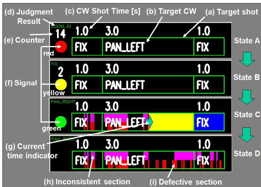
第 9 図 ナビゲーションウィンドウの状態遷移
