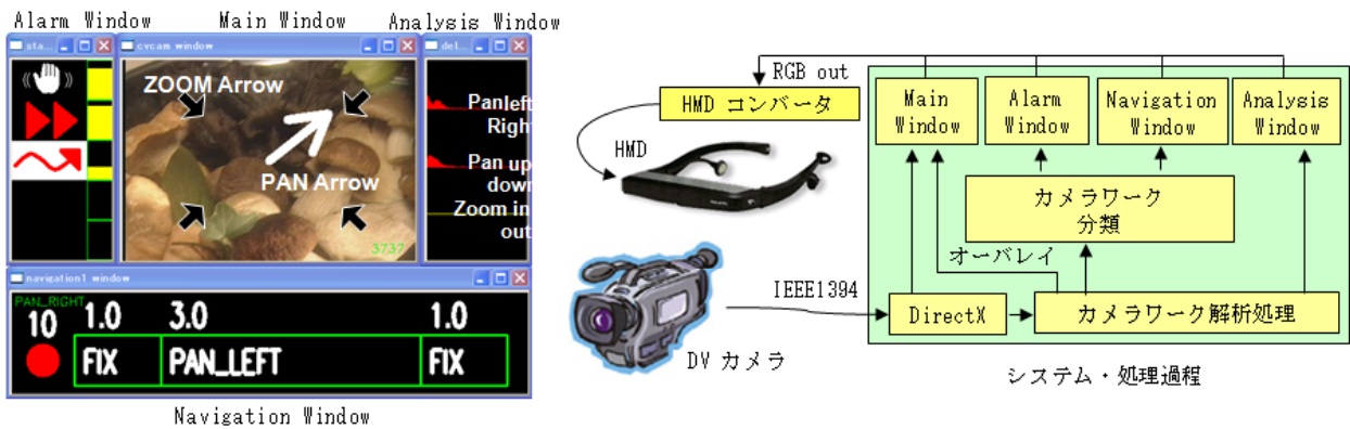
第 8 図 オンライン型映像撮影指南ビデオカメラシステム(プロトタイプ)
