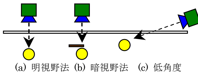
第2図 透過光源を用いた検査光学系の例
