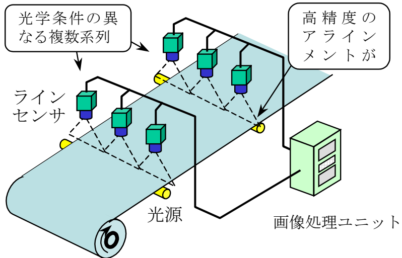
第1図 一般的なウェブ検査システムの構成と問題点
