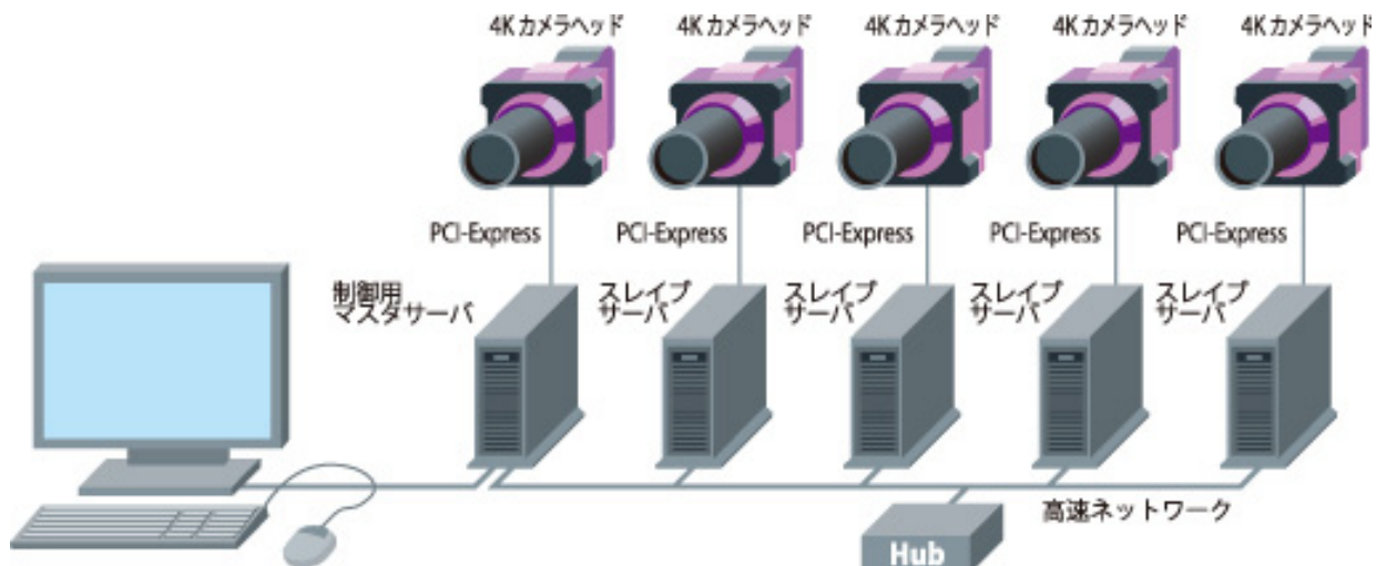
第 2 図 4K カメラヘッドを 5 台用いたマルチカメラシステム“LumiereMulti-5”の構成例
