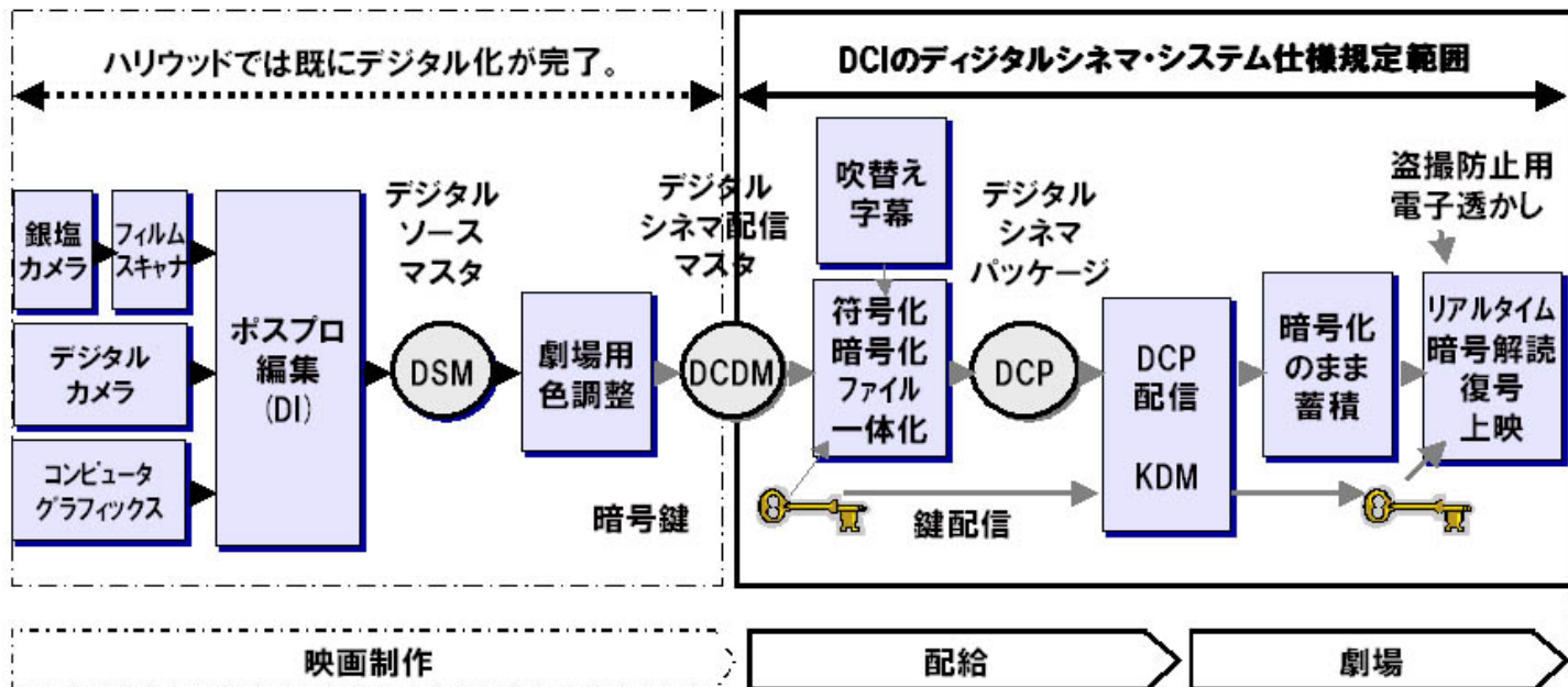
第1図 OCI仕様書が規定するデジタルシネマの配給及びデジタル上映工程
