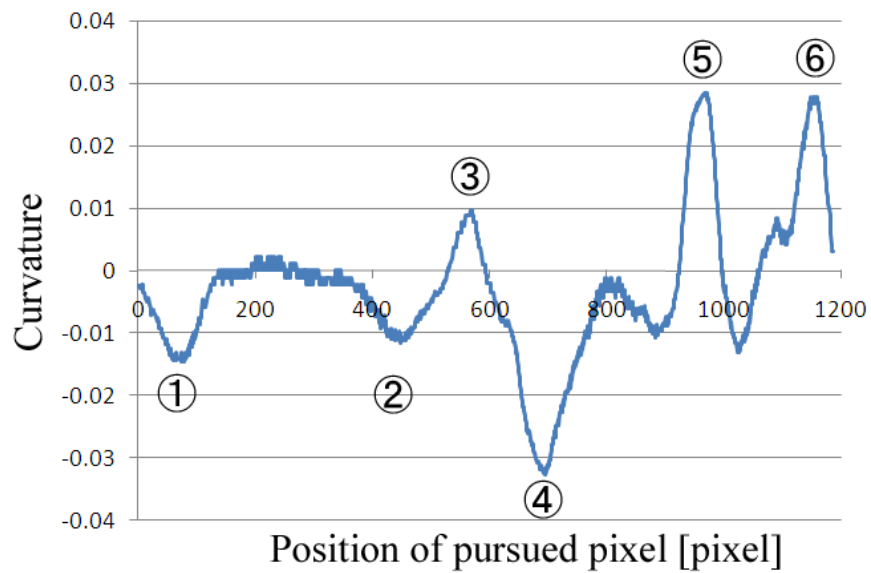
第6図 曲率による指の特徴抽出 (曲率プロフィール)
