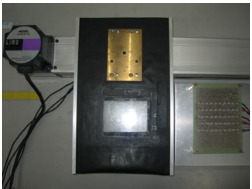
第 9 図 (a) 実験装置全体像 (b) サンプル台と照明装置
