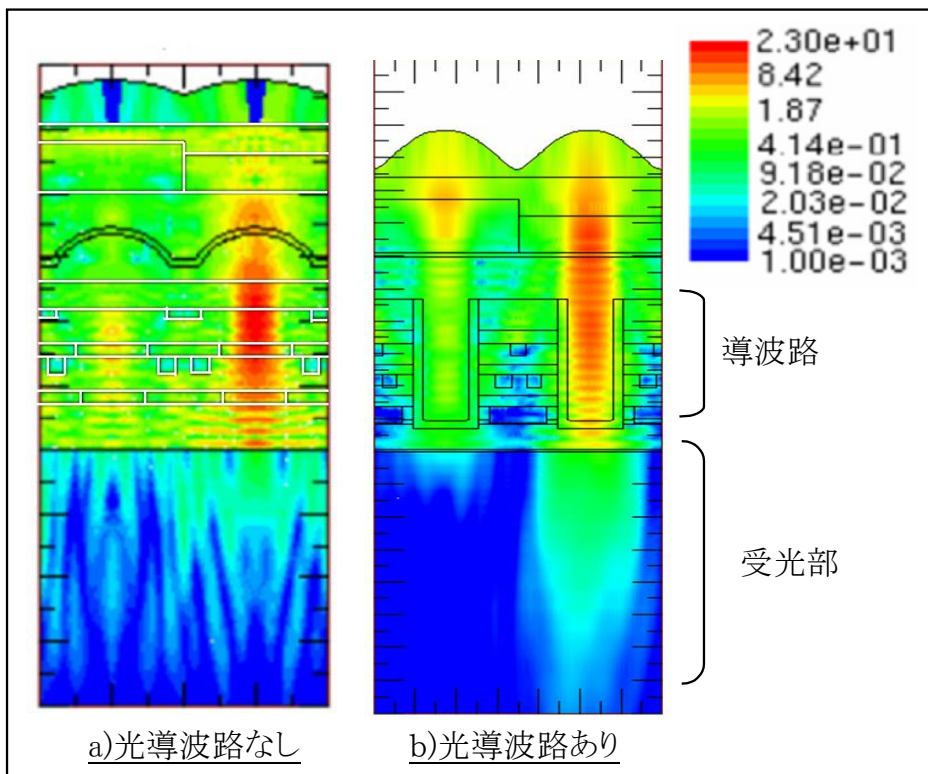
第 10 図 光強度シミュレーション分布
