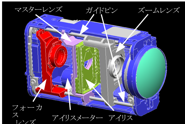
第1図 スリムレンズ
