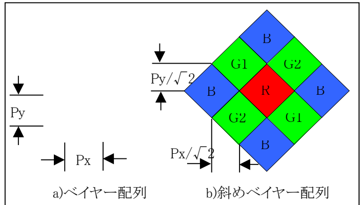
第2図 フィルター構成
