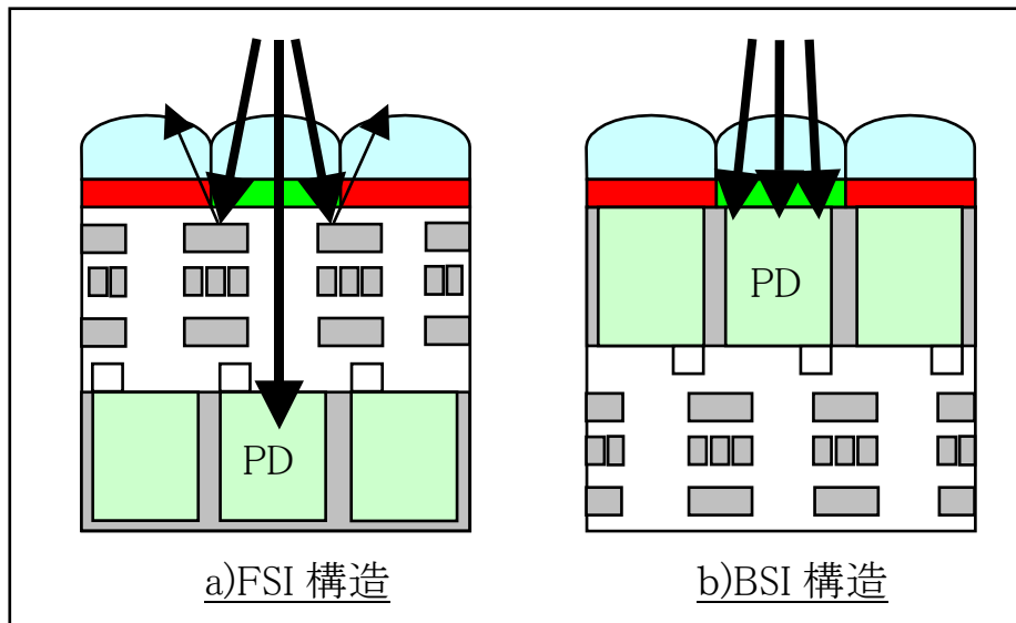
第 9 図 FSI 構造と BSI 構造
