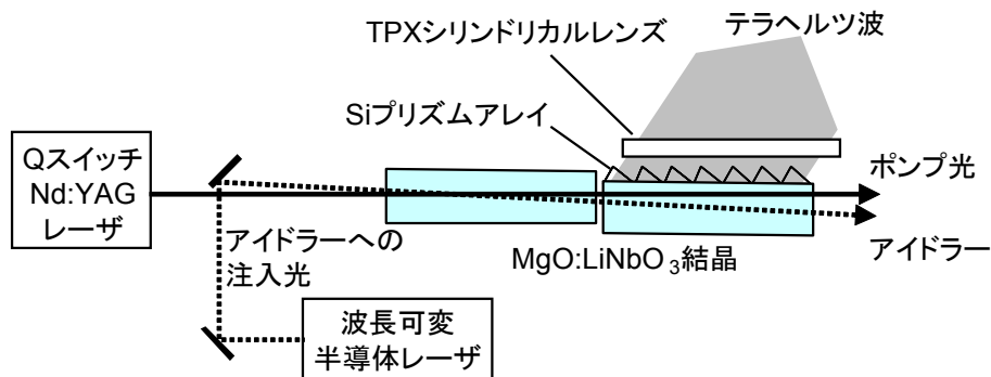
第2図 光注入型テラヘルツ波パラメトリック発生器
