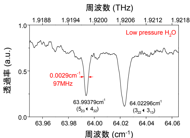
第3図 光注入型テラヘルツ波パラメトリック発生器を用いて測定された水蒸気の吸収スペクトル
