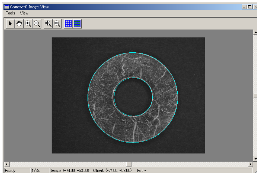
第 5 図 外径・内径の測定結果の画像例（良品）
