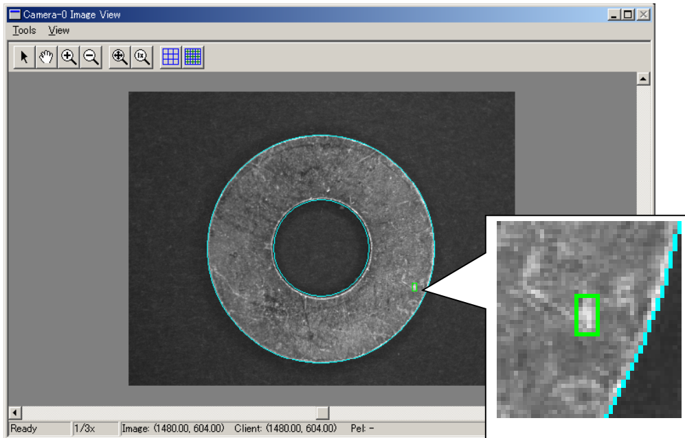
第 4 図 外径・内径の測定結果と検出された欠陥（右の緑四角）
