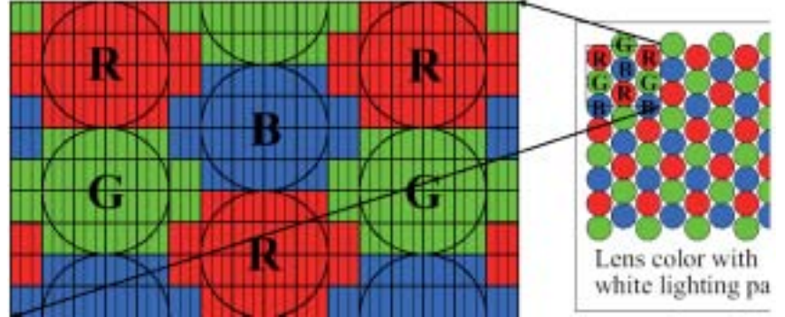
第 3 図 色モアレを防ぐカラーフィルタとレンズ配置
