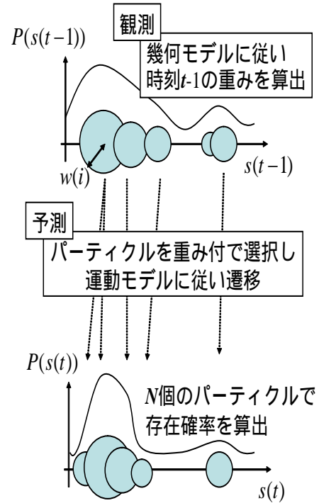
第 2 図 パーティクルフィルタの動作概要
