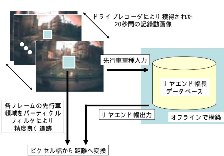
第 1 図 先行車両との車間距離推定
