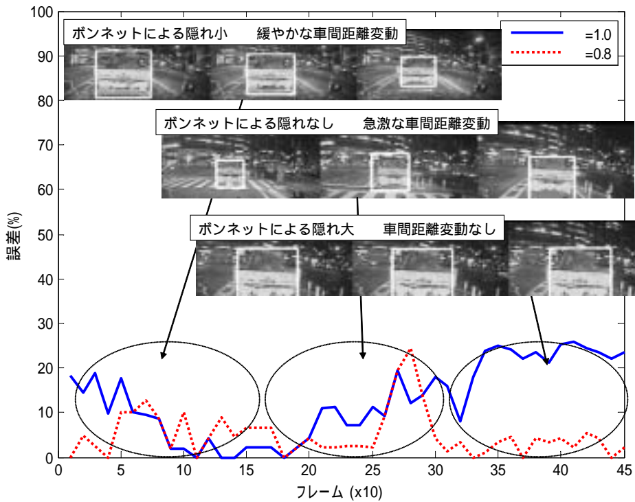
第 4 図 シーケンス 1 におけるリヤエンド幅推定誤差
