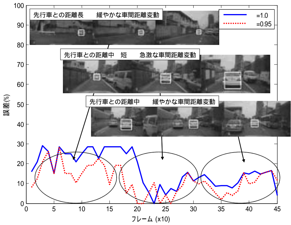
第5図 シーケンス2におけるリヤエンド幅推定誤差
