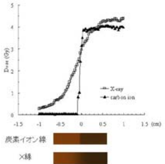
第 4 図 照射野辺縁線量プロファイル
