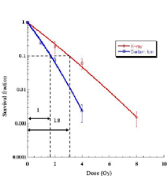
第 3 図 生存率曲線 (A172 細胞)
