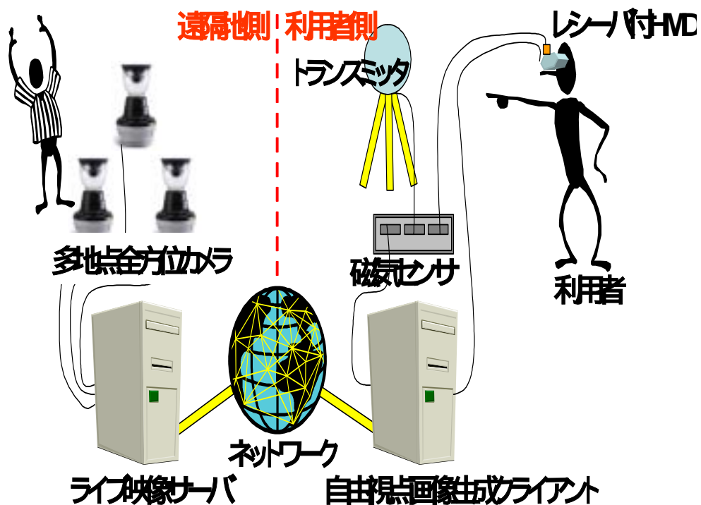
第 2 図 プロトタイプシステムの構成
